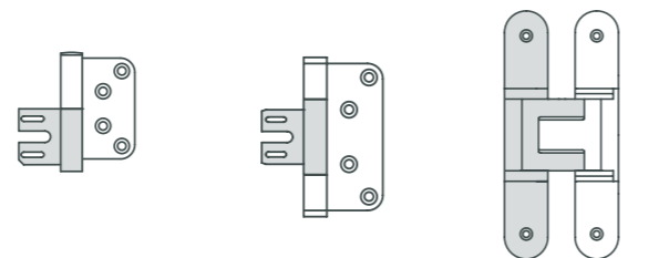
Band V 0080 Rahmenteil V 8100 WF Band V 0087 WF Rahmenteil V 8000 WF Band Tectus TE 340 3D (verdeckt)
